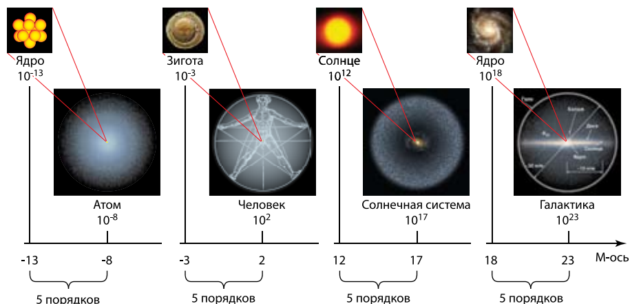
Рис. 34. Структуры типа ядро+оболочка встречаются во Вселенной с определенной периодичностью на масштабной оси 11
