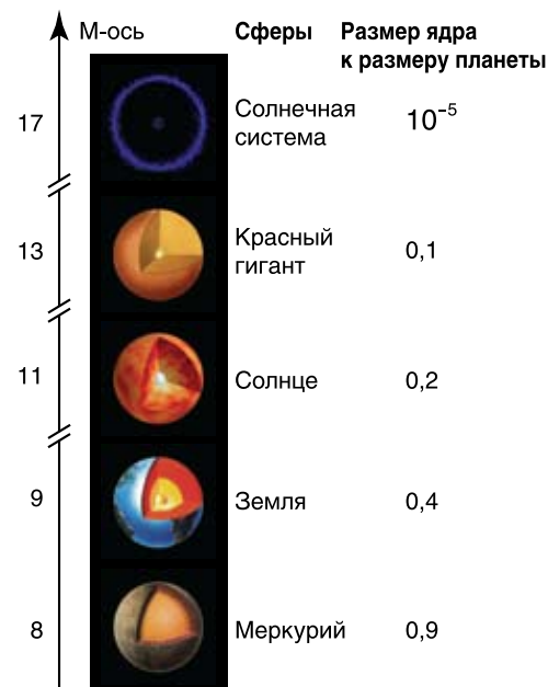
Рис. 35. Принцип яйца — т.е. ядро+оболочки свойственен всем планетам крупнее Меркурия и всем «живым» звездам
