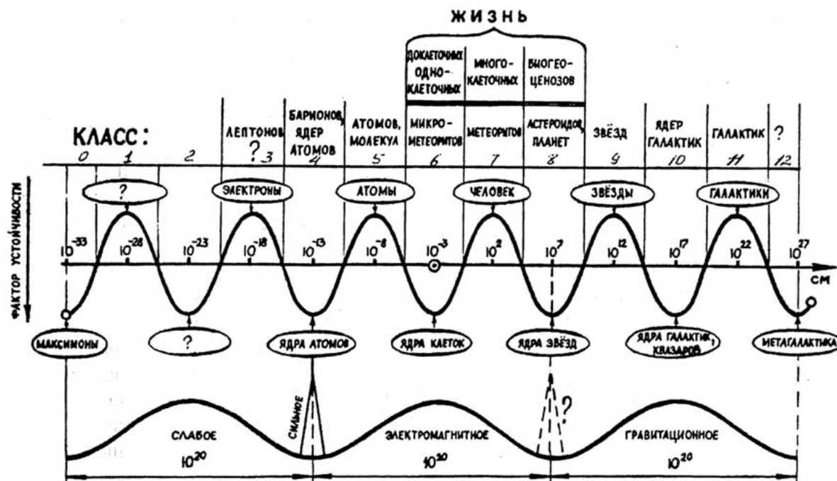
Рис. 1. Все объекты Вселенной расположены вдоль масштабного измерения не случайно и хаотично, а строго упорядоченно и гармонично. Их расположение можно представить в виде синусоидальной волны устойчивости с периодом 10^5 .
