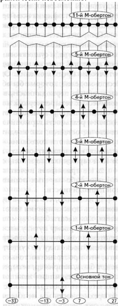
Рис. 22. Гармонические колебания на М-оси (упрощенная модель).
