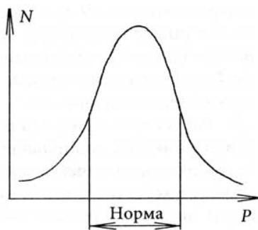
Рис. 16. Нормальное распределение числа объектов N в множестве в зависимости от количества параметров P .
