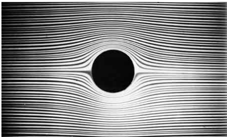
Рис. 43. Ламинарное течение
